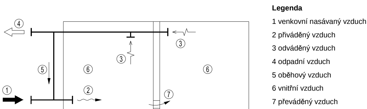
Obrázek 2.2 – Znázornění proudů vzduchu ve větraném prostoru
